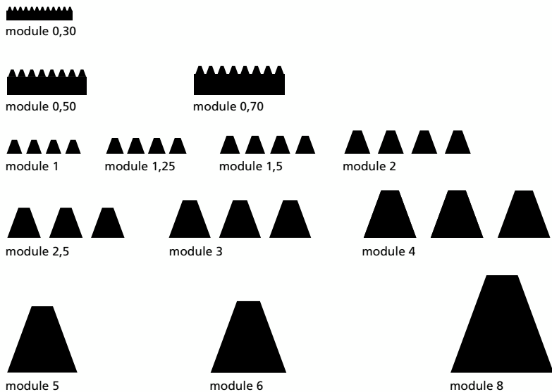
Crémaillères à denture droite - Angle de pression 20°
