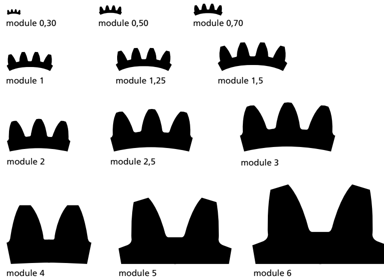
Roues cylindriques droites - Angle de pression 20°
