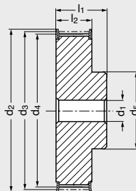
Avec flasques
