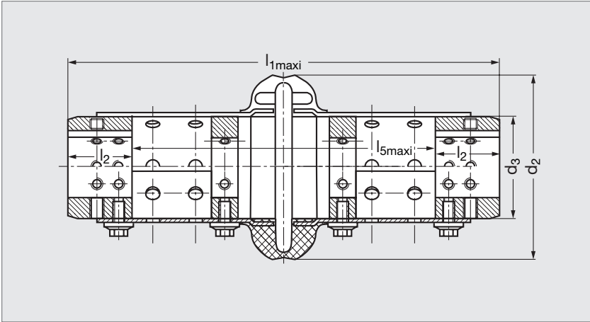
Élément élastique VIVA VSX
